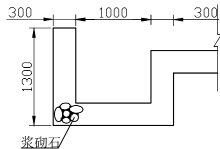
B-B剖面图
