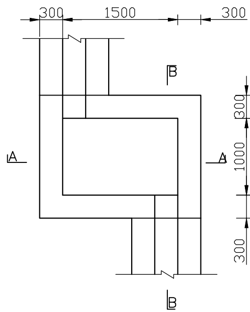
1.5m×1m×1m沉砂池平面设计图
