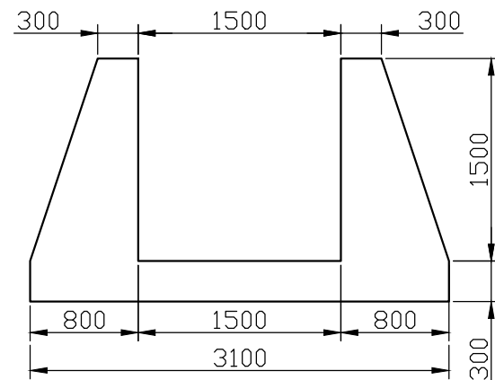
3m×1.5m×1.5m沉砂池C-C剖面图
