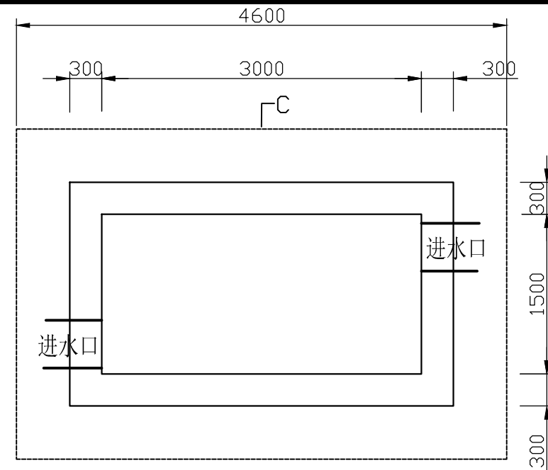
3m×1.5m×1.5m沉砂池平面图
