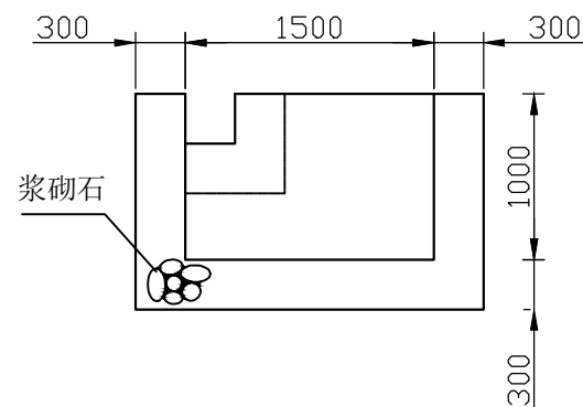
A-A剖面图
